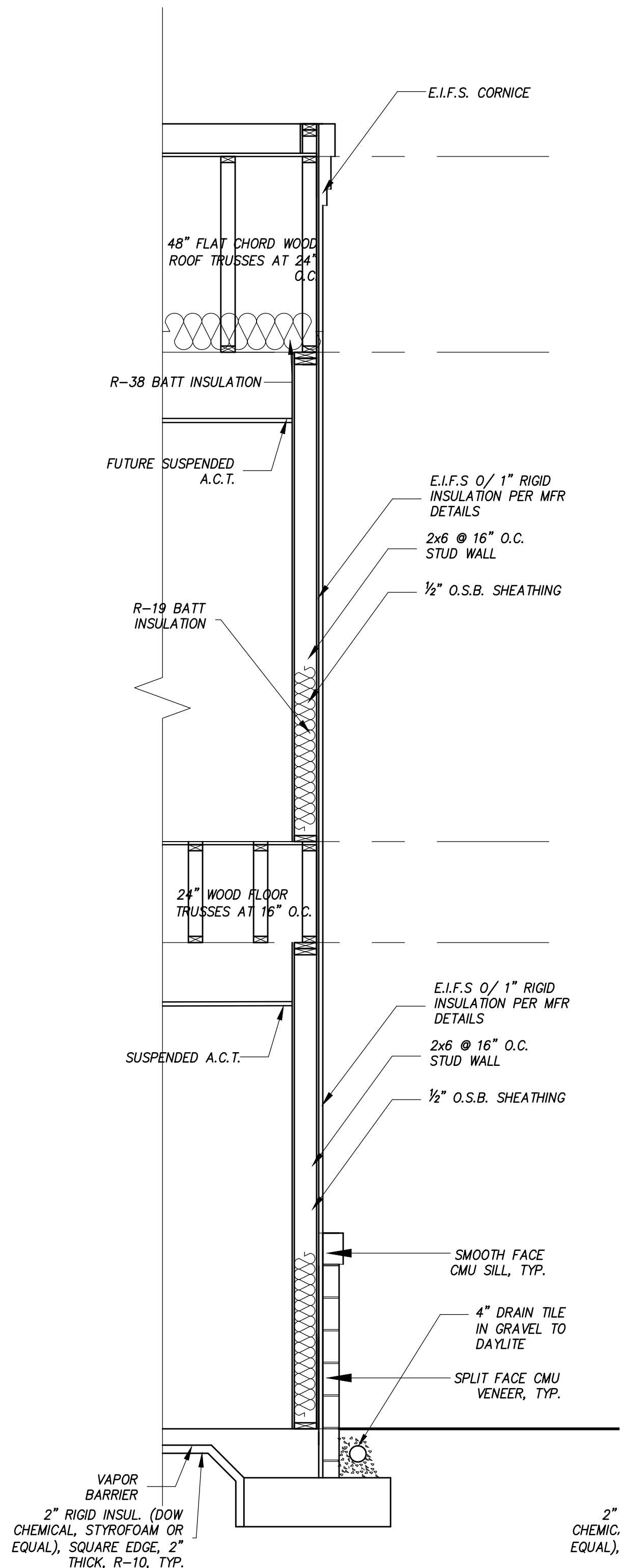
1 WALL SECTION A9 SCALE: 1/2"=1'-0"
