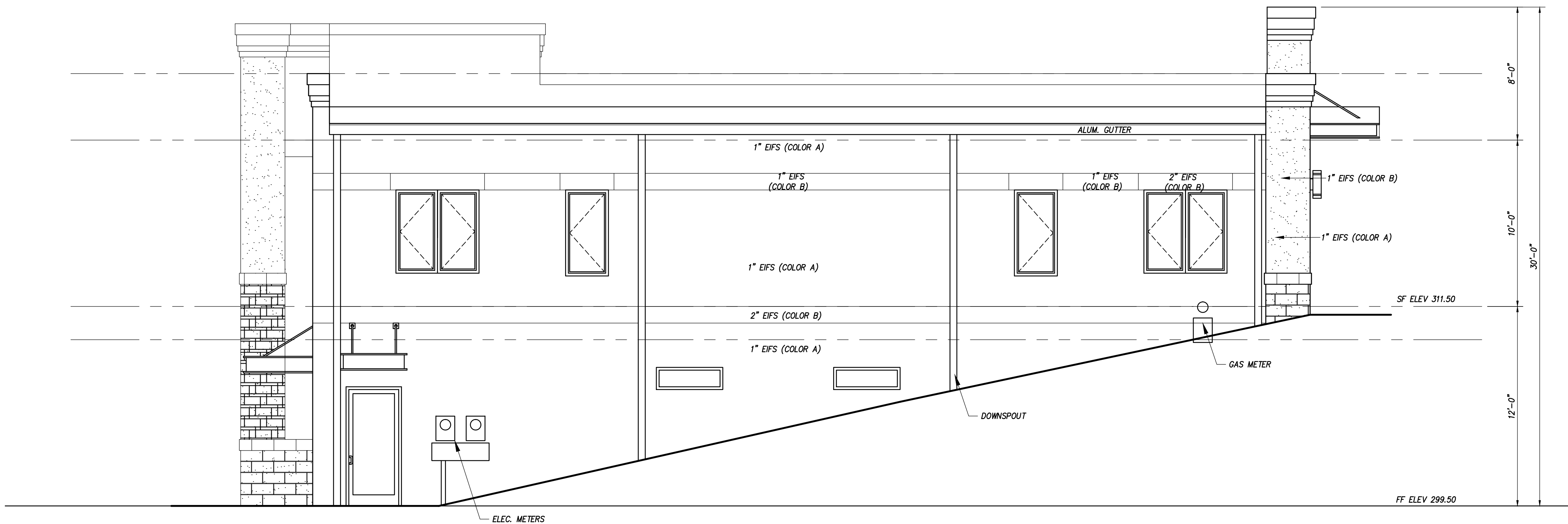
RIGHT ELEVATION
