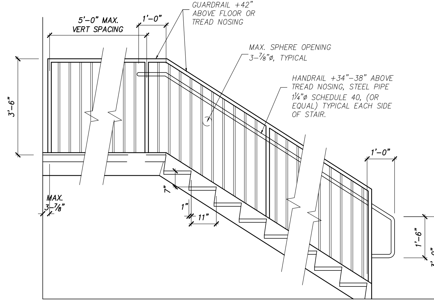
2 STAIR DETAIL A11 SCALE: 3/4"=1'-0"
